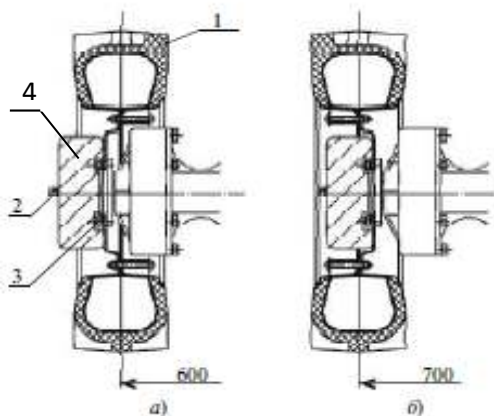
Рисунок 2.4 - Схема регулировки колеи мотоблока
