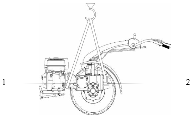
Рисунок 2.1 –Схема строповки мотоблоков «New Sich MB»
