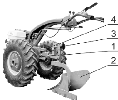
Рисунок 3.1 - Мотоблок в агрегате с плугом
