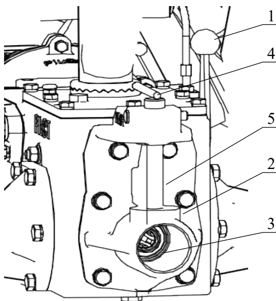
Рисунок 1.5 –Сцепка ВОМ
