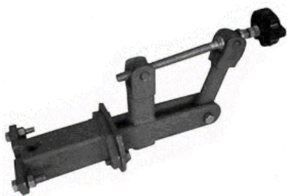
Рисунок А 1 – Сцепка для мотоблока МТЗ №6
